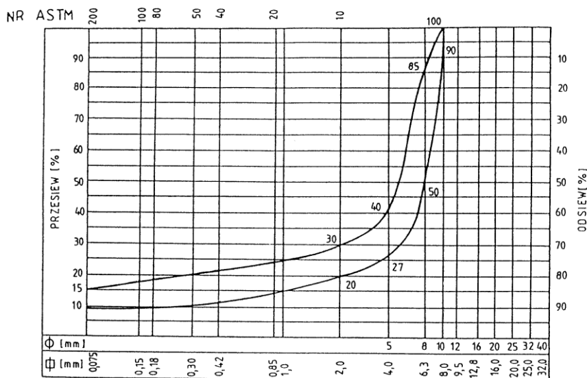
Rys. 3. Krzywe graniczne uziarnienia mieszanek mineralnych SMA od 0 mm do 8 mm
