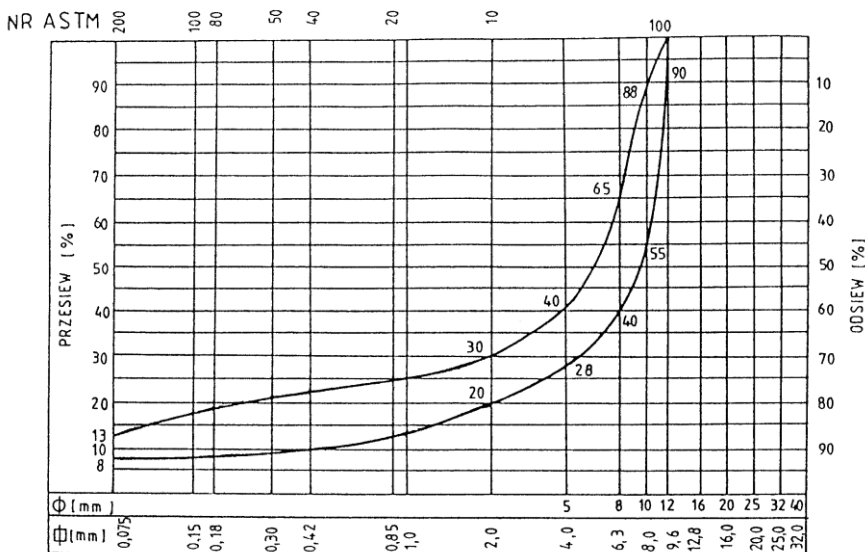
Rys. 4. Krzywe graniczne uziarnienia mieszanek mineralnych SMA od 0 mm do 9,6 mm
